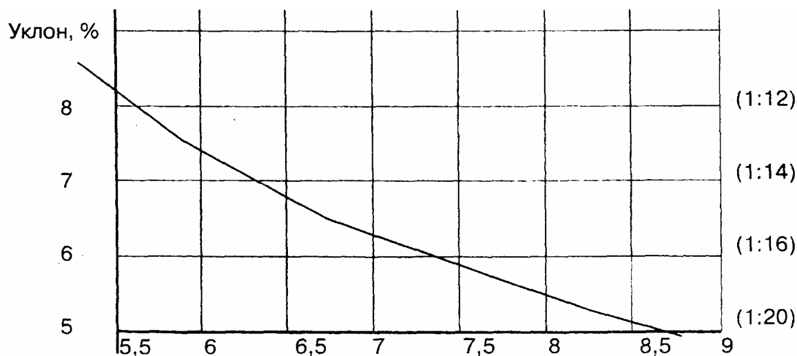
Минимальный внутренний радиус винтового пандуса, м Рисунок 8.1 — Зависимость внутреннего радиуса винтового пандуса от величины его уклона
